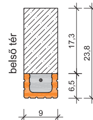
19. Leier MDA nyílásáthidaló elhelyezési lehetőségei
