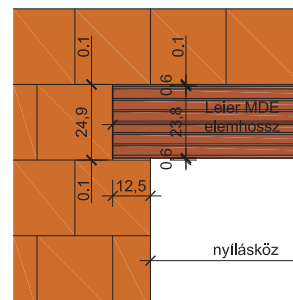
42. Méretek – Leier MDE nyílásáthidaló
