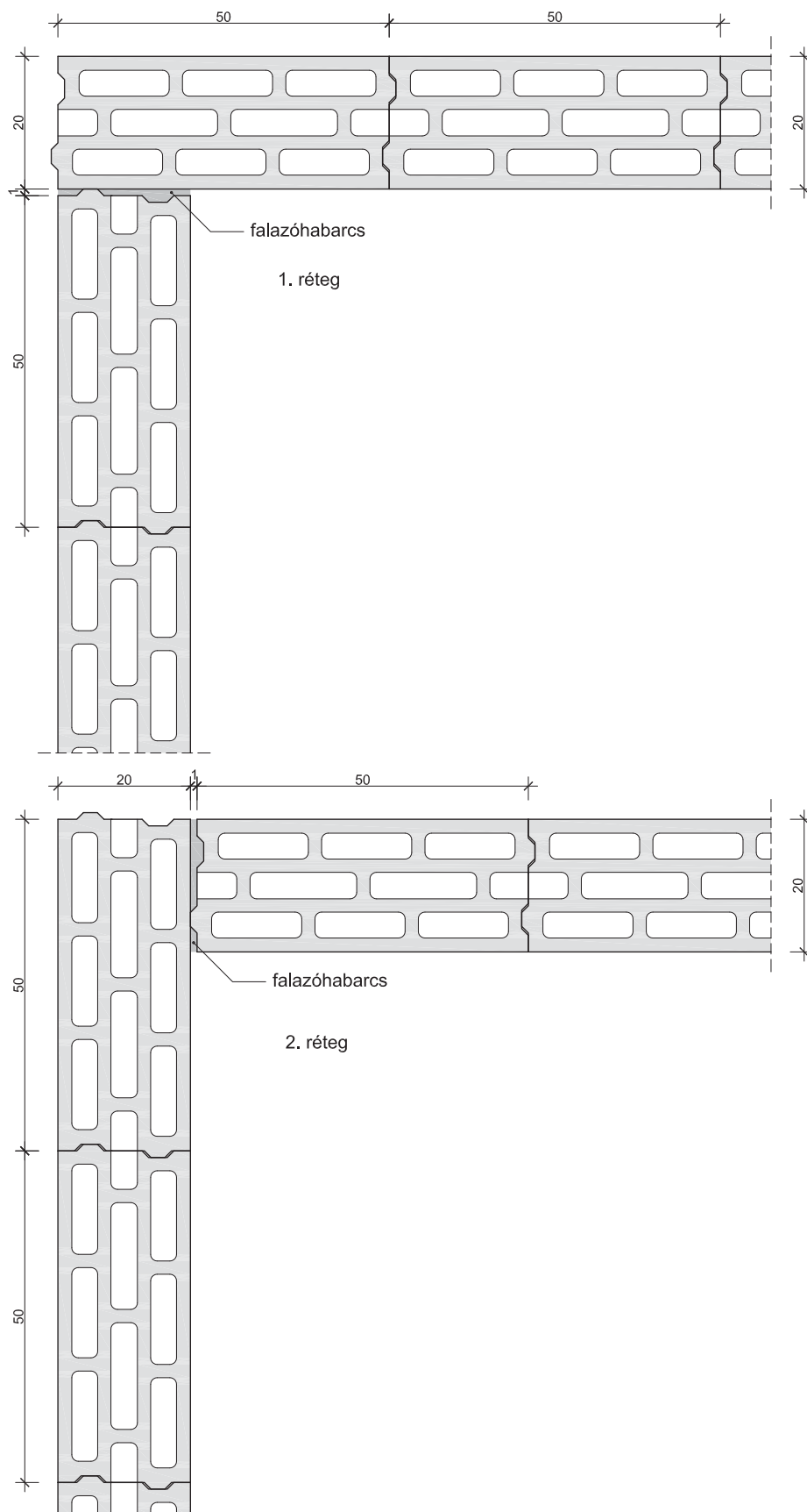
20. Falsarok: Leier beton főfalelem FF 20
