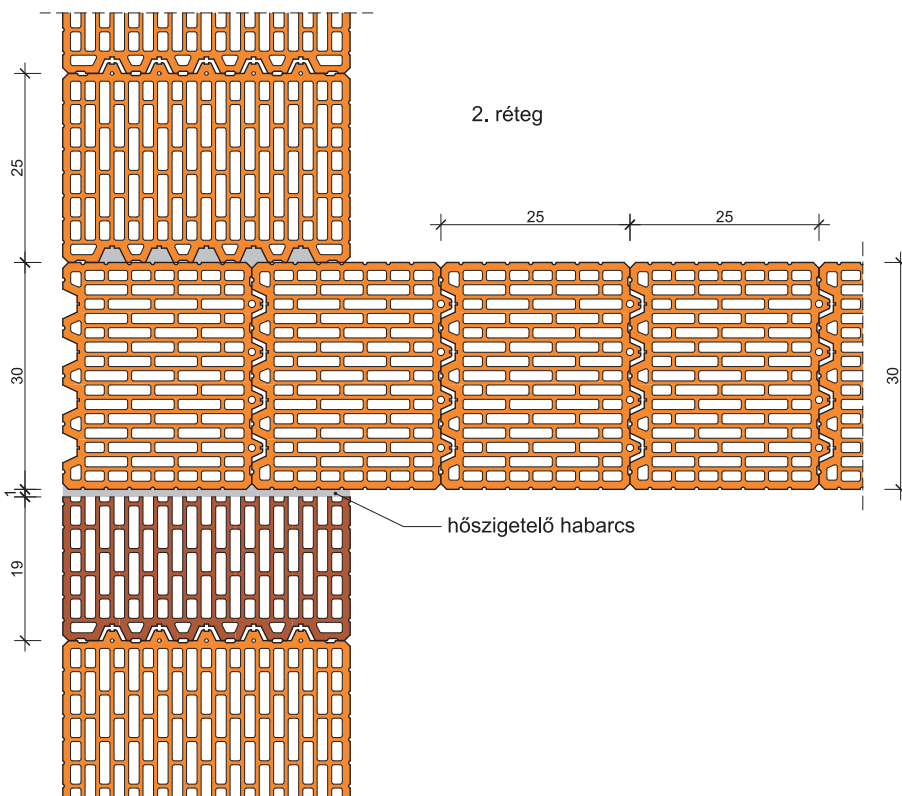
74. Falcsatlakozás: LeierPLAN 38 Pro – LeierPLAN 30 Pro / LeierPLAN 38 N+F – LeierPLAN 30 N+F Leiertherm 38 Pro – Leiertherm 30 Pro / Leiertherm 38 N+F – Leiertherm 30 N+F
