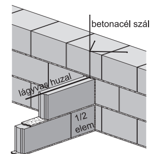
2. Beton válaszfal csatlakozása főfalhoz
