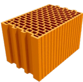
Leiertherm 25 N+F
