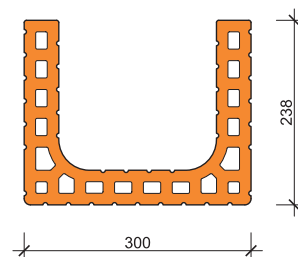
22. Leiertherm 30 U koszorúelem metszete
