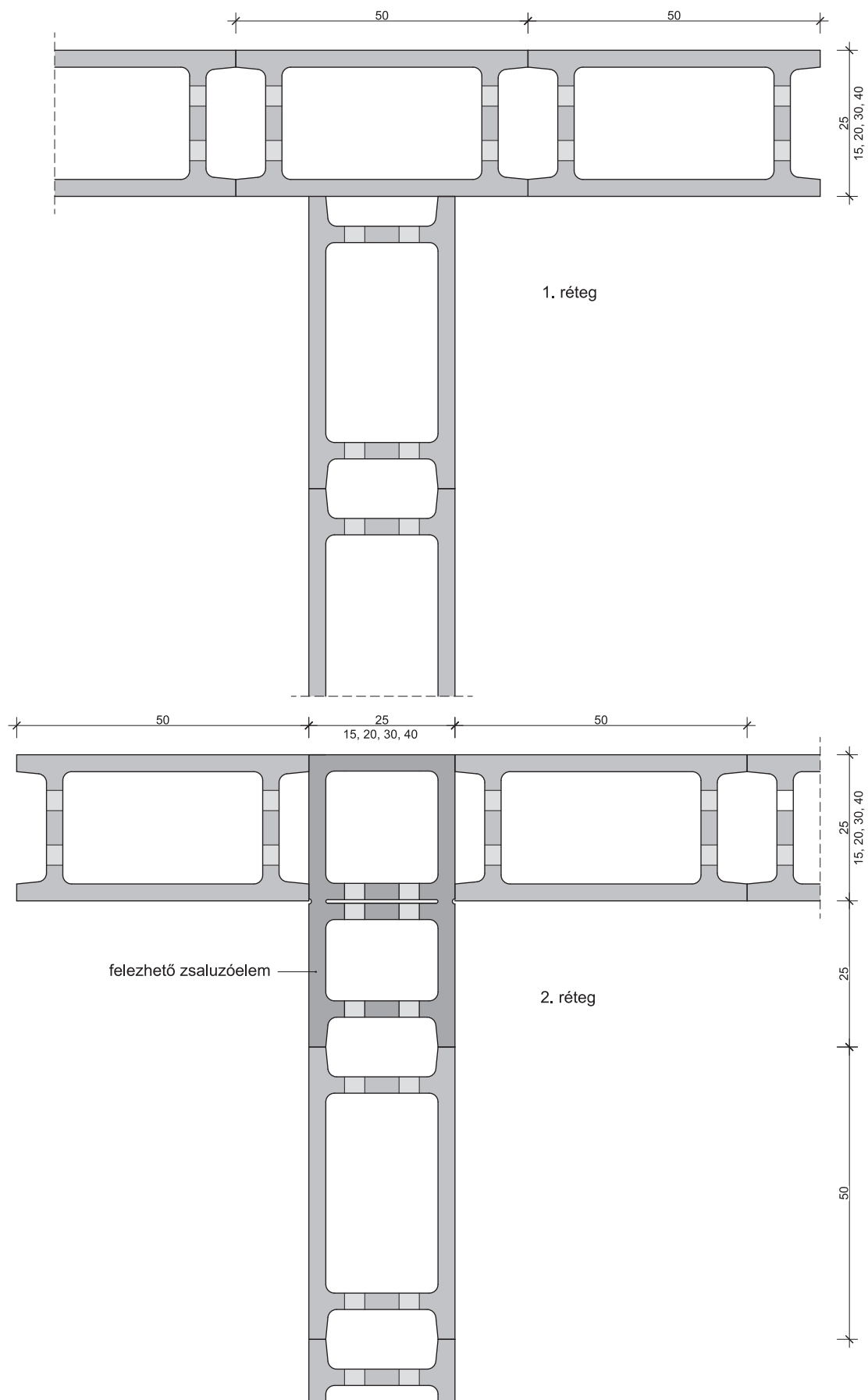
21. Falcsatlakozás: Leier beton zsaluzóelem (ZS 15, ZS 20, ZS 25, ZS 30, ZS 40)
