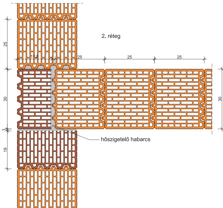
71. Falcsatlakozás: LeierPLAN 30 Pro – LeierPLAN 30 Pro / LeierPLAN 30 N+F – LeierPLAN 30 N+F Leiertherm 30 Pro – Leiertherm 30 Pro / Leiertherm 30 N+F – Leiertherm 30 N+F
