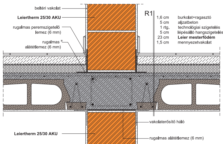
40. Hanggátló fal és földem kapcsolata
