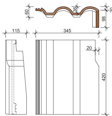
jobbos szegélycserep
