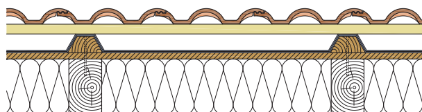
3. Vízzáró alátétszigetelés
