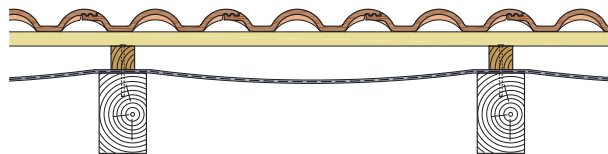
1. Szabadon fekvő alátétfedés
