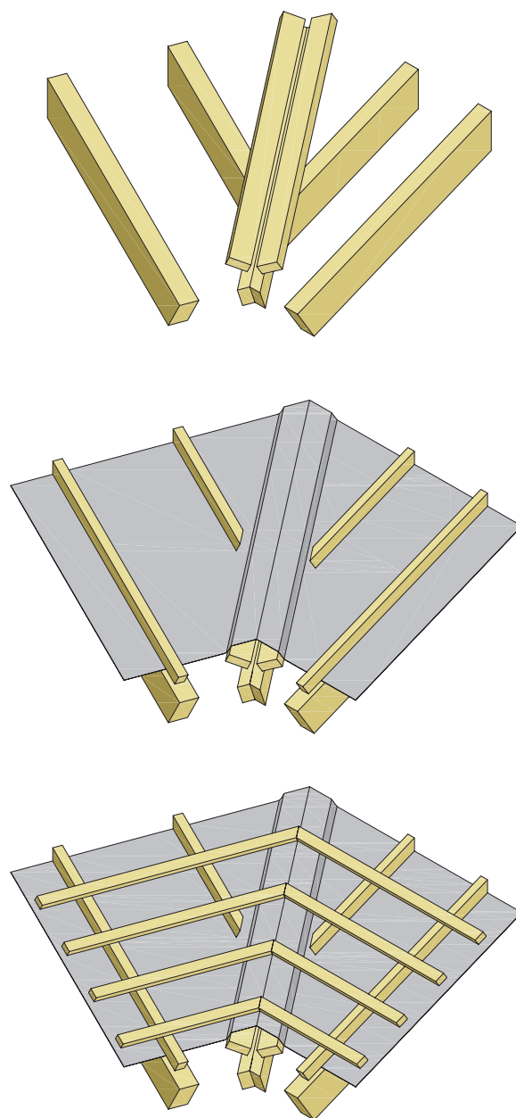
5. Alátétthéjazat vápánál
