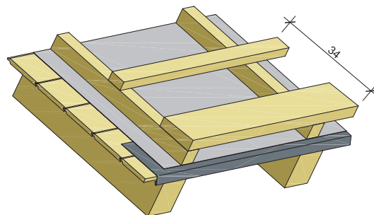
2. Ereszpalló elhelyezkedése – Toscana fedésnél
