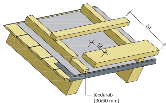
3. Ereszpalló elhelyezkedése – Granite fedésnél
