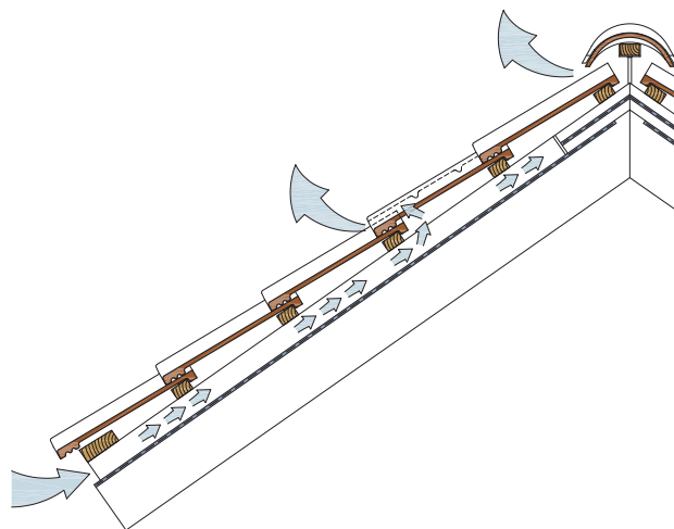
11. Tető átszellőzése
