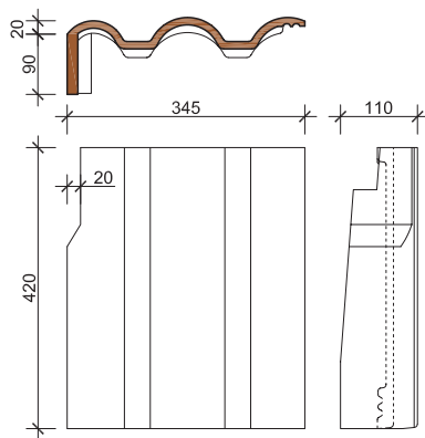
balos szegélycserep
