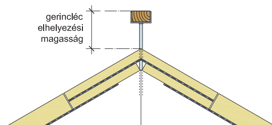
6. Gerincléc elhelyezési magassága – Toscana
