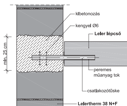
10. Leier lépcső „fészkelése” kerámiafalba
