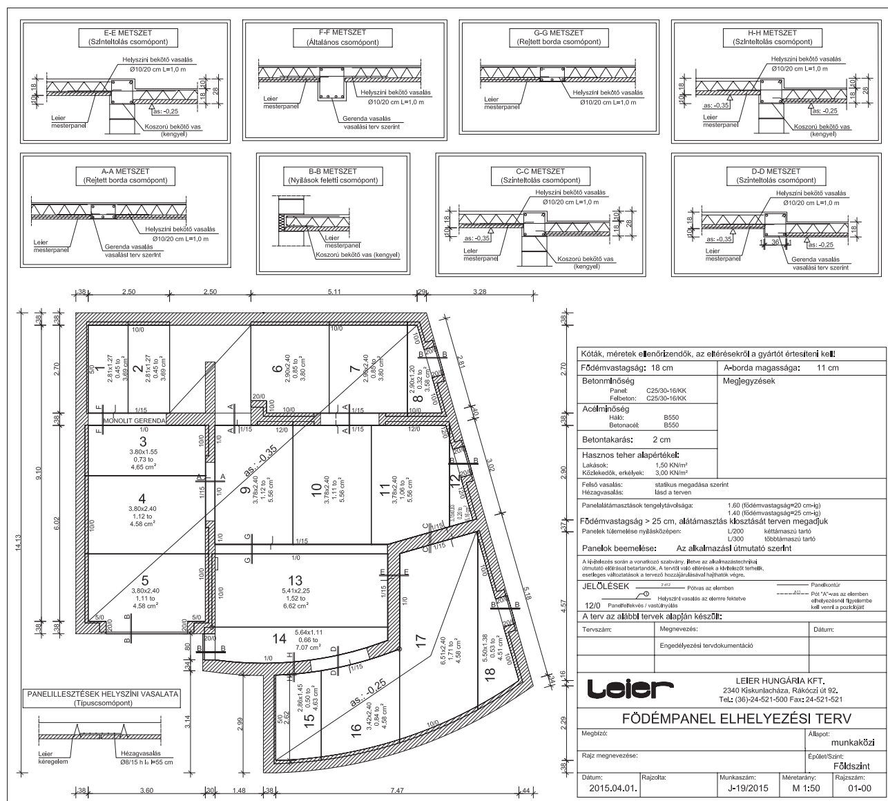
10. Leier mesterpanel (LMP) – Födémpanel elhelyezési terv
