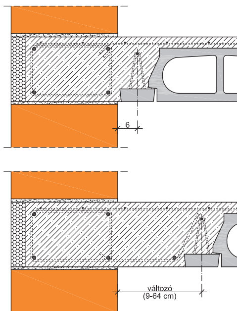
9. Leier mesterfödém szélső födémmezője
