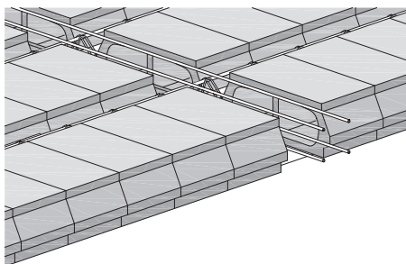
6. A keresztgerenda kialakítása Leier mesterfödém
