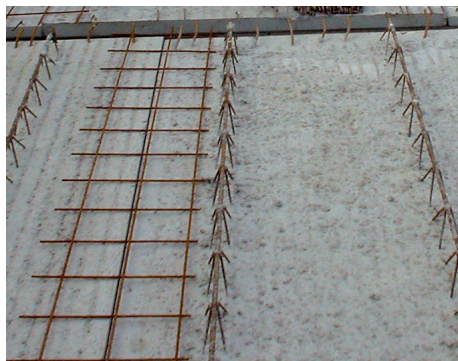
22. Elosztóvasalás Leier mesterpanelek (LMP) között
