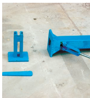
24. Támasztóoszlop, oszloptartó csomópont, feszítőék
