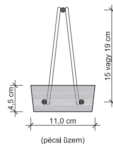
2. Leier mesterfödém gerenda (LMF)
