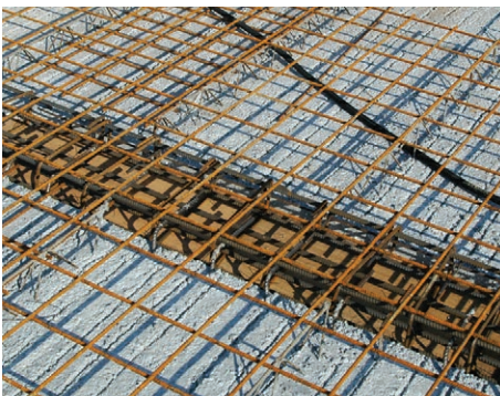
26. Áthidalás feletti vasalás
