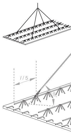
19. Mesterpanel emelése
