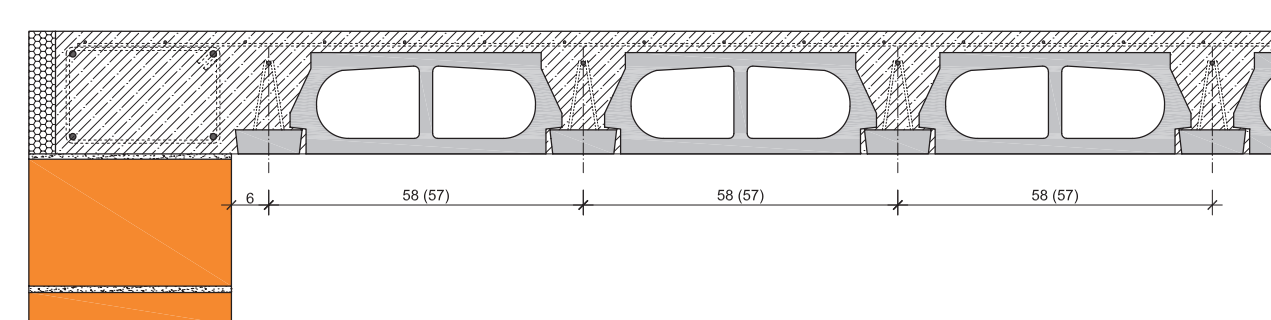
8. Leier mesterfödém, kiosztási méretek
