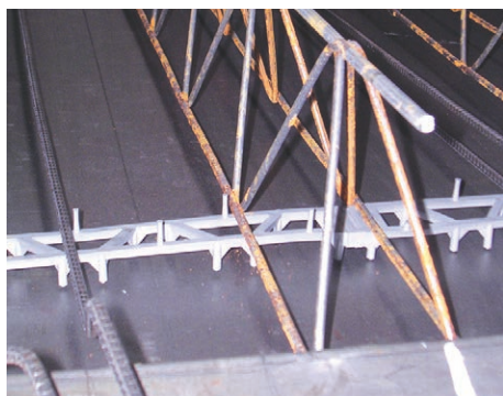
2. Leier mesterpanel (LMP) vasalása
