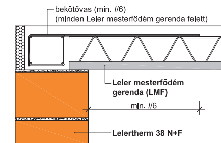
5. vas Leier mesterfödém
