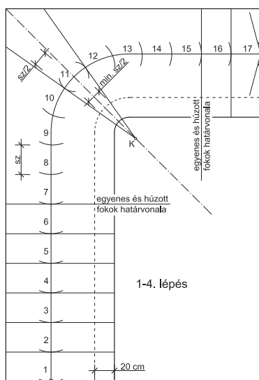
11. Húzott karú lépcső (90°, L alakú) szerkesztése
