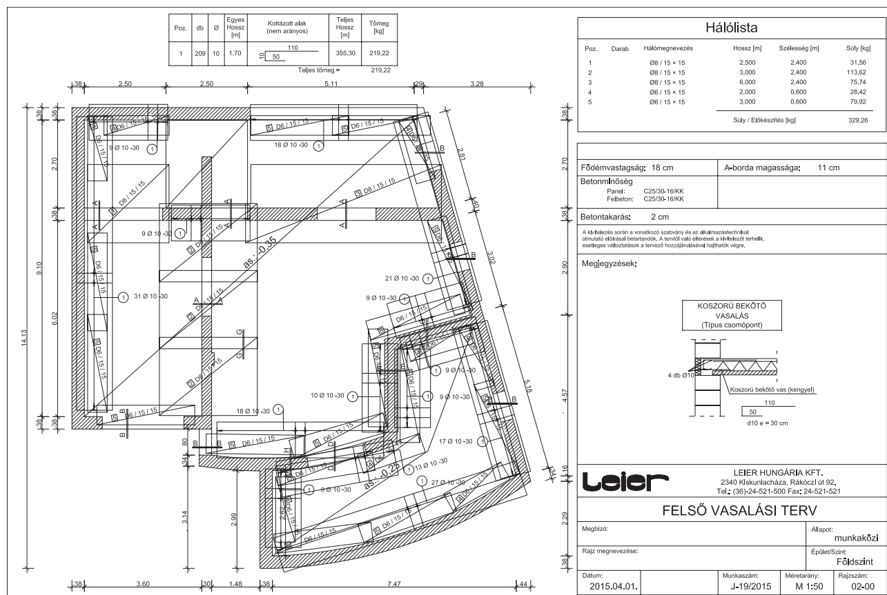
11. Leier mesterpanel (LMP) – Felső vasalási terv
