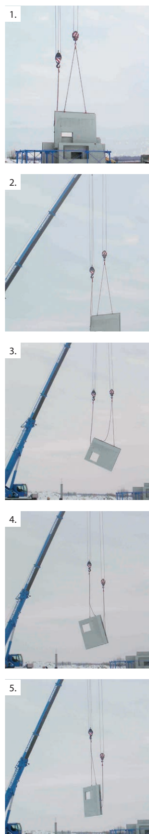
32. Leier kéregfal (LKF) levegőben történő forgatása
