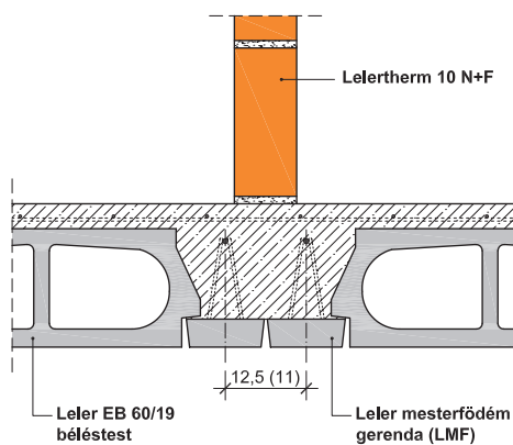
10. Válaszfal alatti gerendakettőzés Leier mestergerendákkal (LMF)
